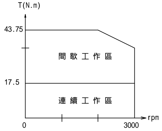
MA2-5500M
