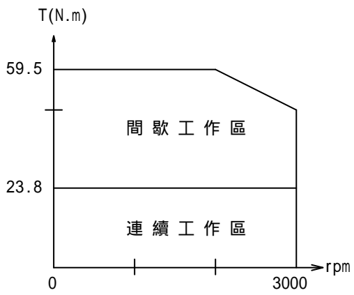
MA2-7500M
