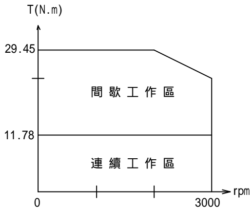
MA2-7500M
