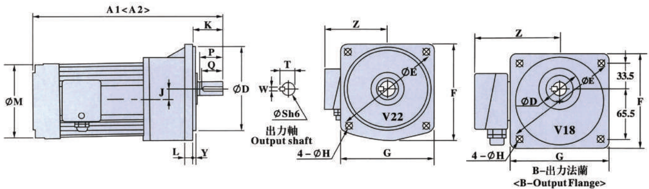
尺寸表(m/m)
