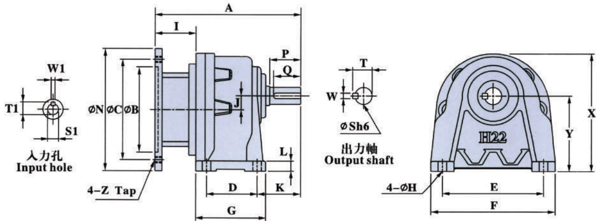
尺寸表(m/m)
