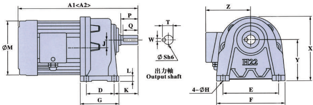
尺寸表(m/m)
