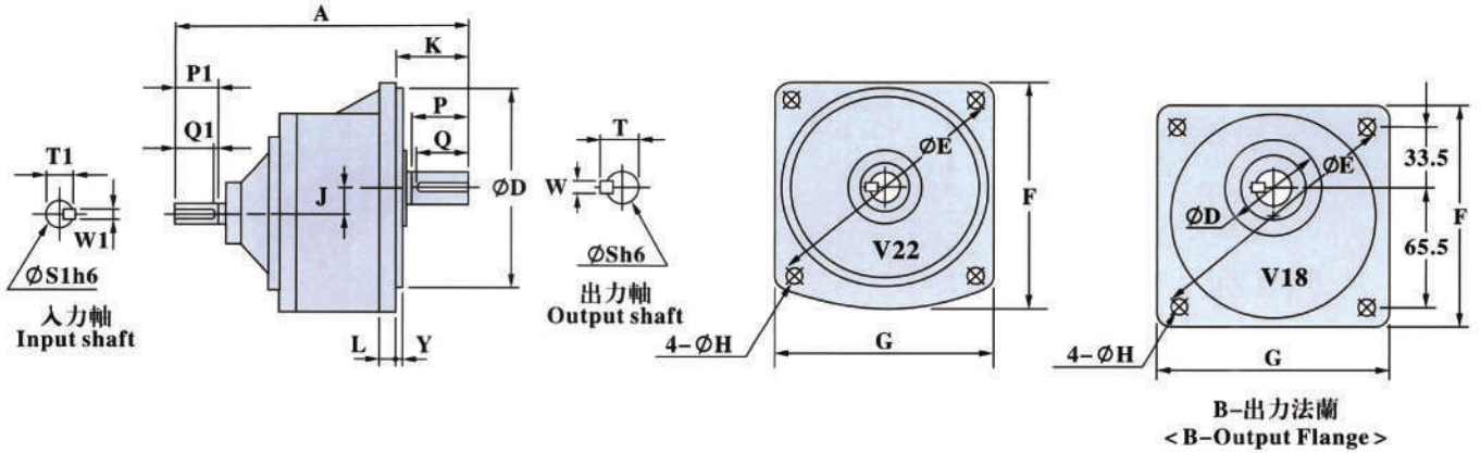
尺寸表(m/m)
